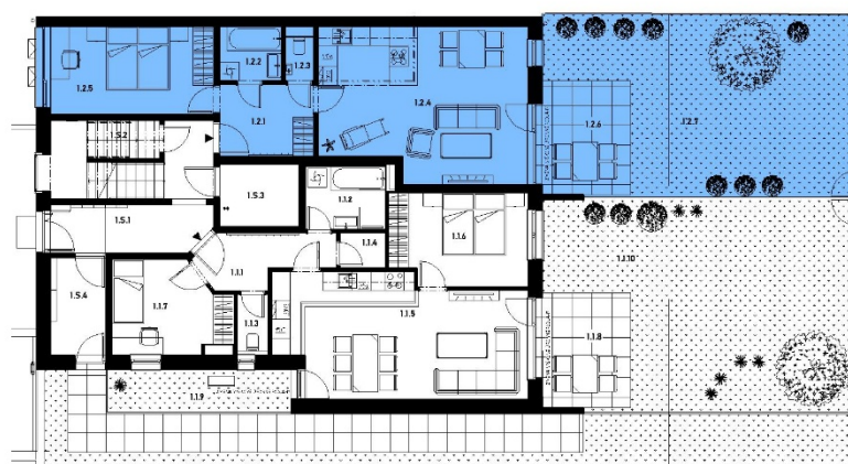
PŮDORYS 1.NP
