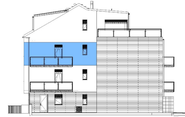
JIŽNÍ POHLED
